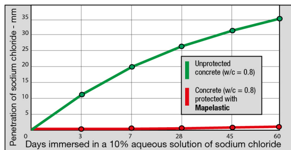
Fig. 3: Beskyttelse med Mapelastic mod indtrængning af natriumklorid i porøs beton
