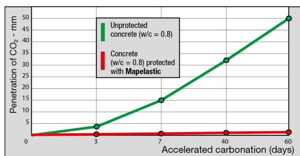
Fig. 2: Beskyttelse med Mapelastic mod accelereret karbonatisering (30 % CO 2 ) af porøs beton
