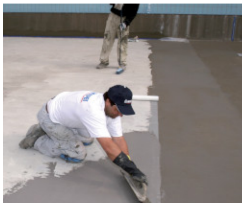
Vandtætning af et svømmebassin med Mapelastick
